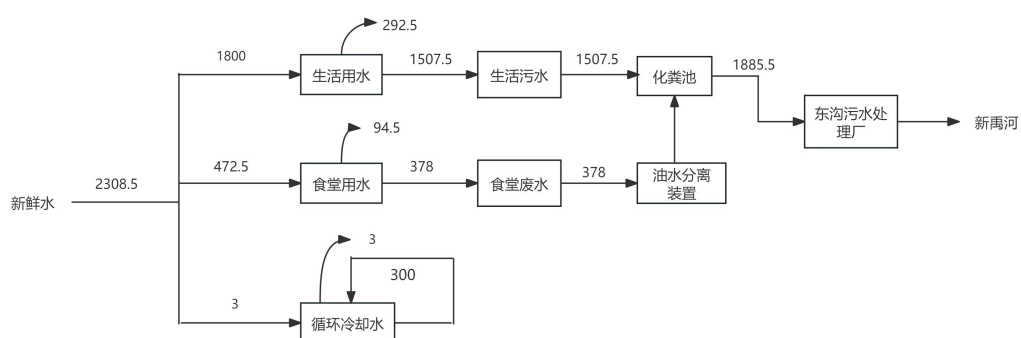
图 2-2 改扩建后全厂水平衡图 单位：t/a
