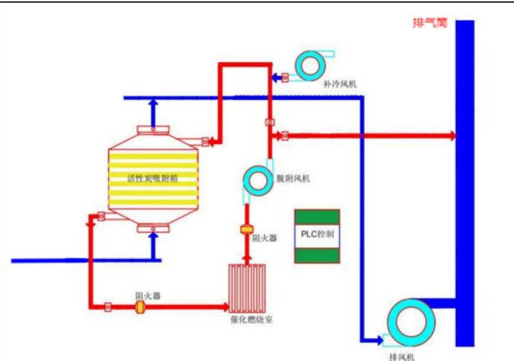
图 4-2 活性炭吸附+催化燃烧装置工艺流程图
