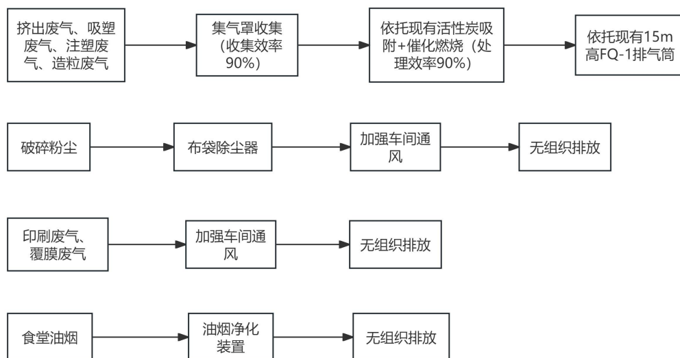
图 4-1 废气收集治理工艺流程图
